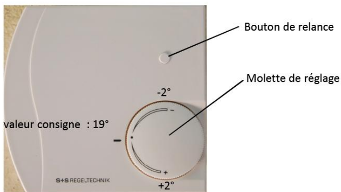
Sonde d'ambiance
